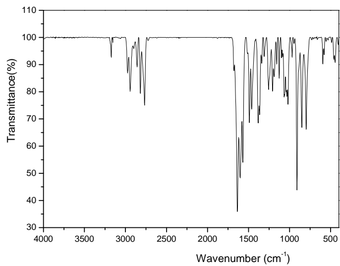
Fig. 1S IR spectrum of HL.
